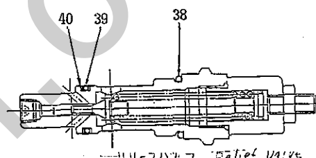
リリーフバルブ Relief Valve
