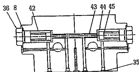
B-B 断面 SECTION B-B
